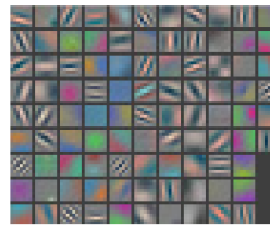
(b) ZFNet
